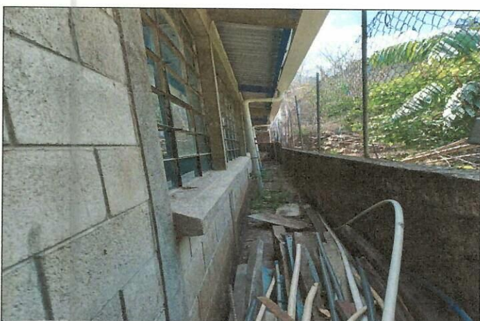
Foto 3: Se realizará reforzamiento del muro de contension, debido a que no se encuentra reforzado ni en buenas condiciones, ocasionando que se incline hacia el establecimiento.
